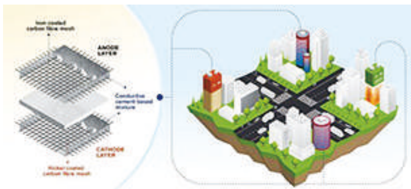
▲新發明以水泥製作的電池示意圖。
